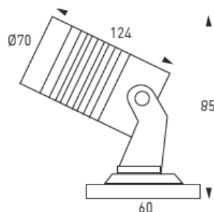
GLS15W(CCT)IP65
